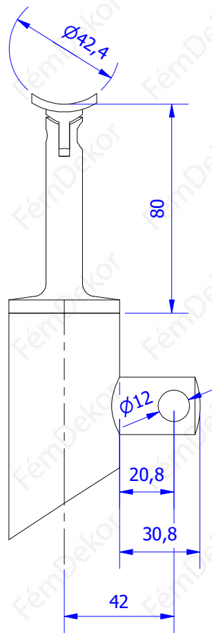
F-F (1 : 2)
