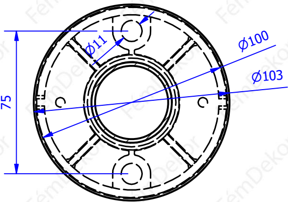
D-D ( 1 : 2 )
