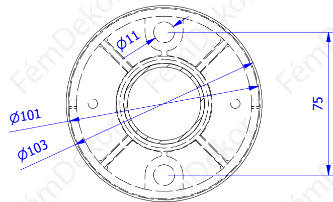
A-A ( 1 : 2 )
