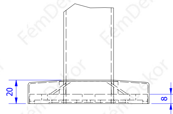
B ( 1 : 2 )
